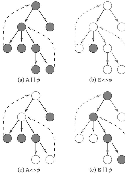
Fig. 17. (T)CTL-formulae
